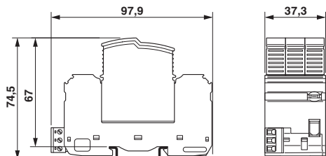
Dessin coté
